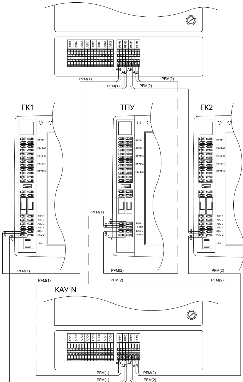
Рисунок 10 – С резервированием по интерфейсу PFM
