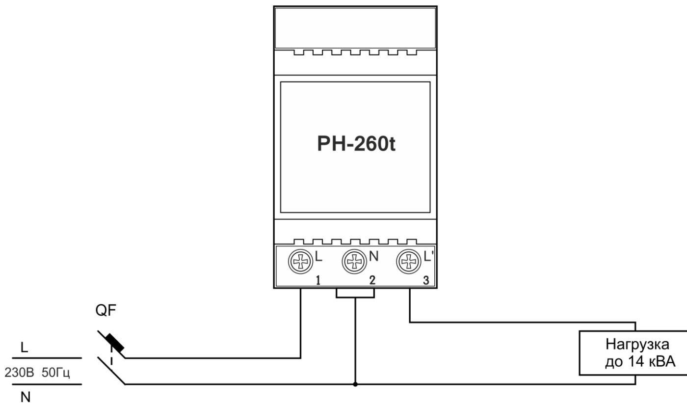
Рисунок 2 – Схема подключения изделия
