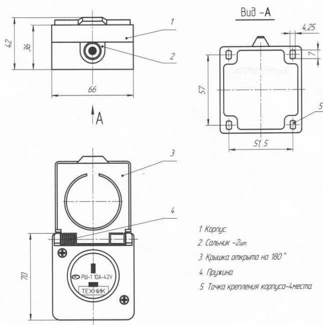
Розетка РШ-1-10А-42V
