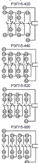
Схемы электрические принципиальные реле и ограничителей перенапряжений
