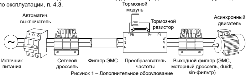
Рисунок 1 – Дополнительное оборудование
