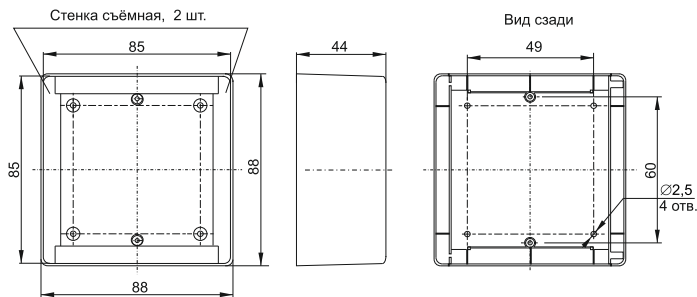
Рисунок 2 – КМКУ артикул СКК10D-U-1-KXX
