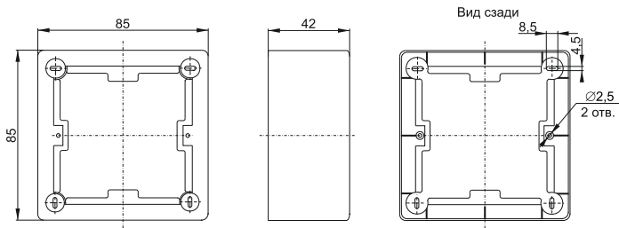
Рисунок 1 – КМКУ артикул СКК10D-U-2-KXX
